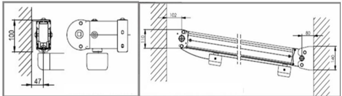
montaż rozpórkowy
